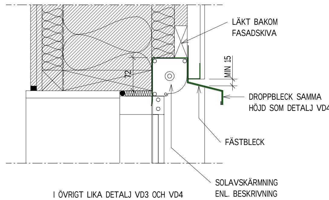
EV1 PRINCIP ELEVATION 1:10 RULLSKIFTS BALK - MED BYGEL
