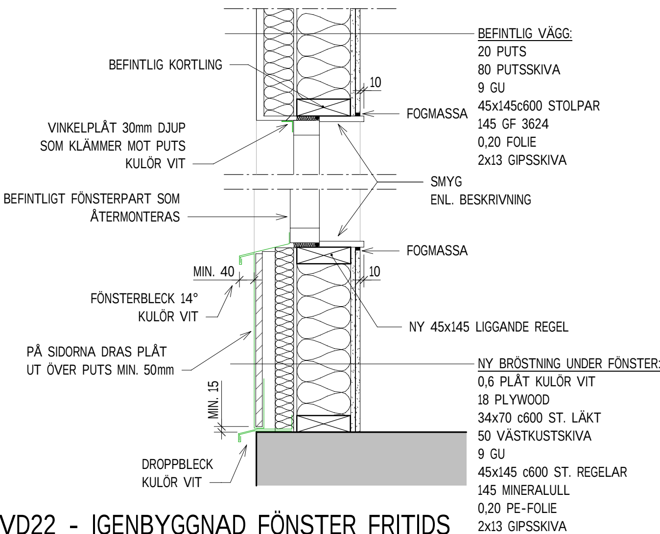
VD22 - IGENBYGGNAD FÖNSTER FRITIDS 1:10
