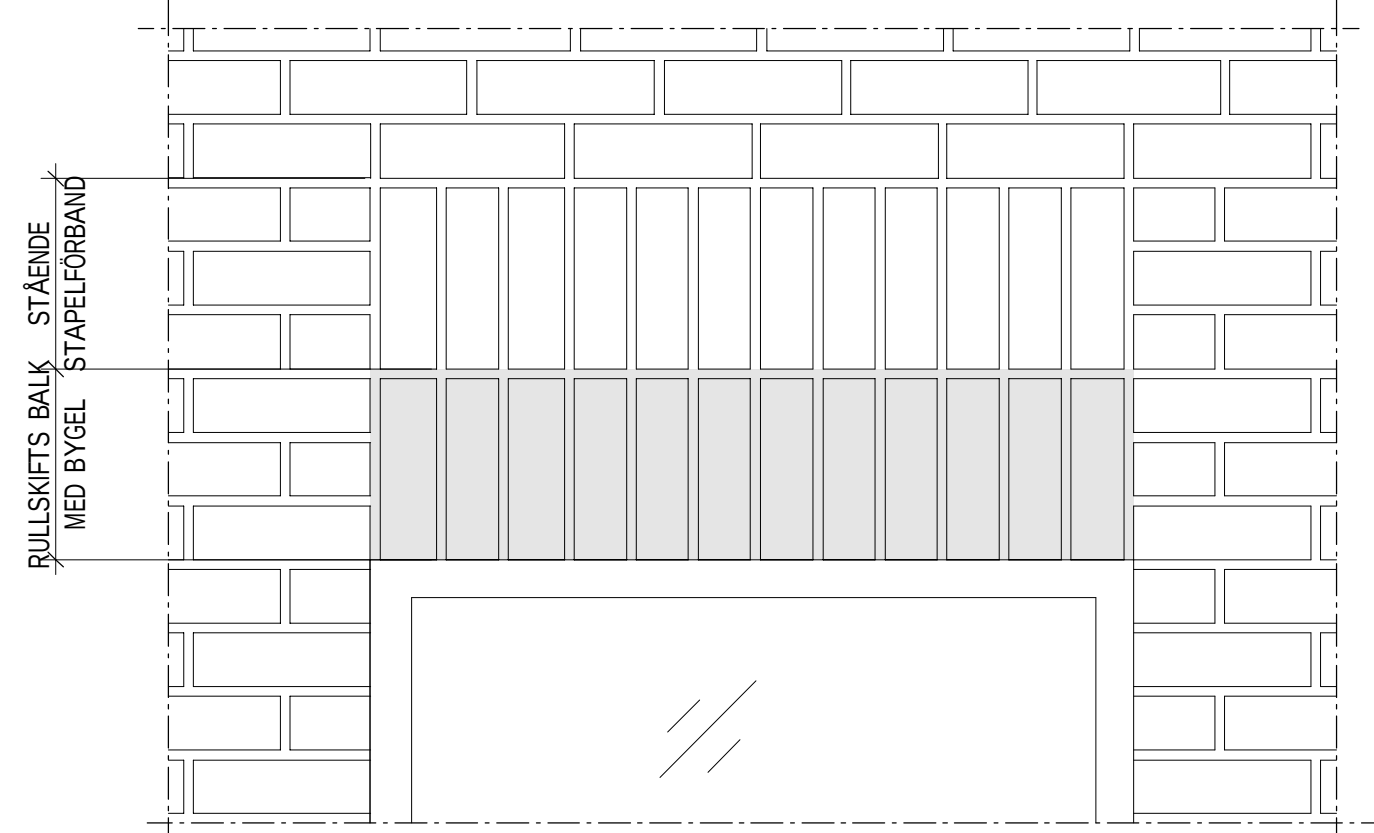
EV1 PRINCIP ELEVATION 1:10 RULLSKIFTS BALK - MED BYGEL
